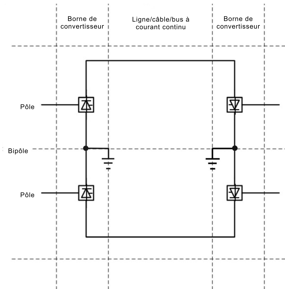
Figure 2 – Structure du système CCHT
