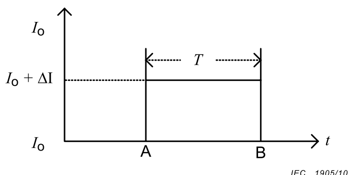
Figure 9 – Essai de réponse indicielle de la commande de courant au niveau de l'onduleur
