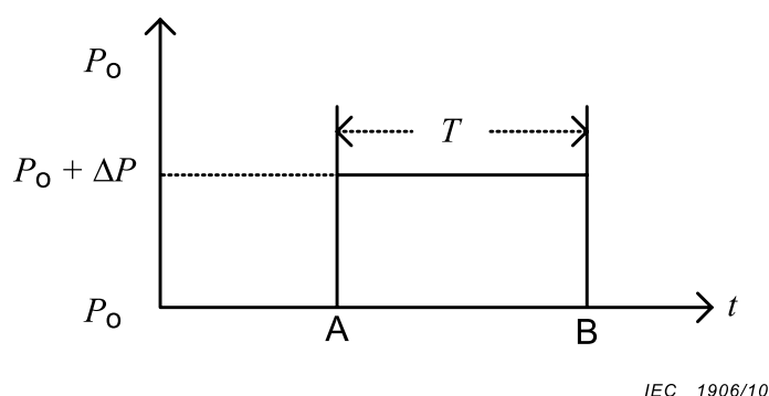
Figure 10 – Essai de réponse indicielle de la commande de puissance au niveau du redresseur
