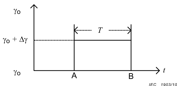
Figure 7 – Essai de réponse indicielle de la commande d'angle d'extinction au niveau de l'onduleur
